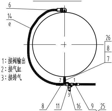
Трубопровод тормоза хода 盘式制动器接管示意图
