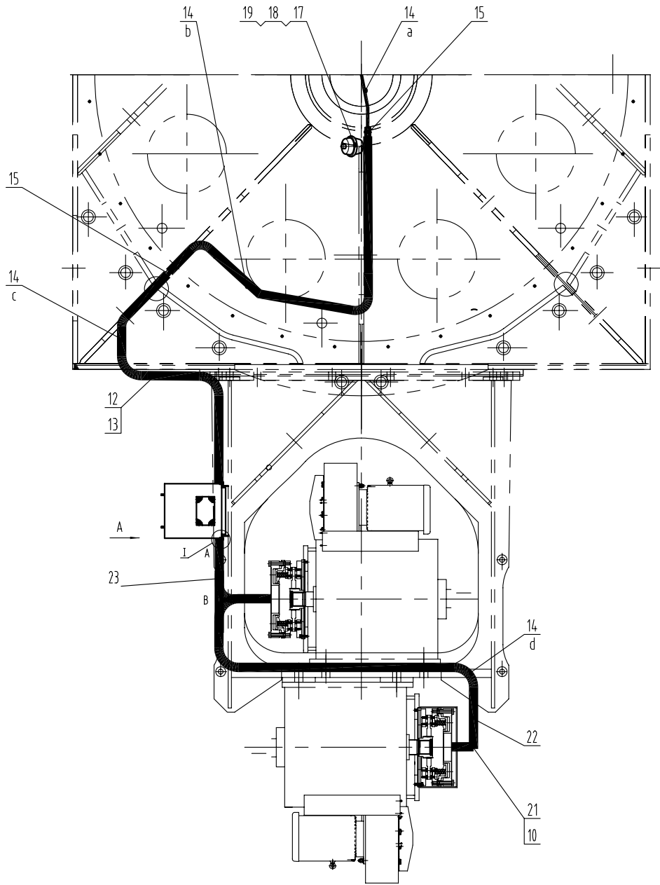
Трубопровод тормоза хода 盘式制动器接管示意图
