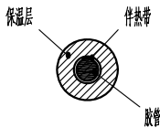
其他段件热保温示意图
